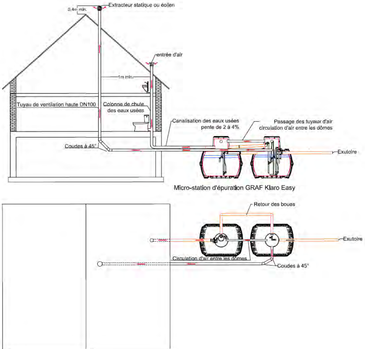
Illustration 11 : ventilation Easy
