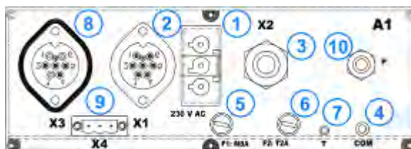
Illustration 4 : vue arrière de l'automate
